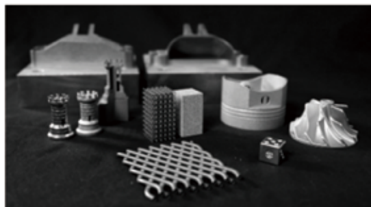
金属 3D プリンタにより作製した造形物
